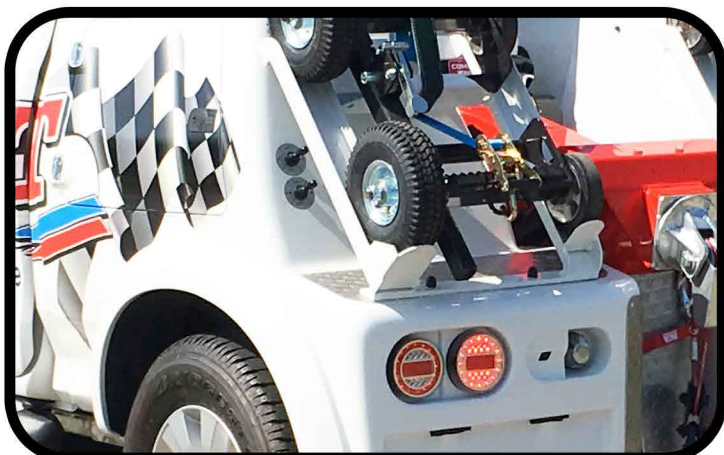
- Deux manipulateurs pour les fonctions du bras et du treuil en complément de la commande radio.
