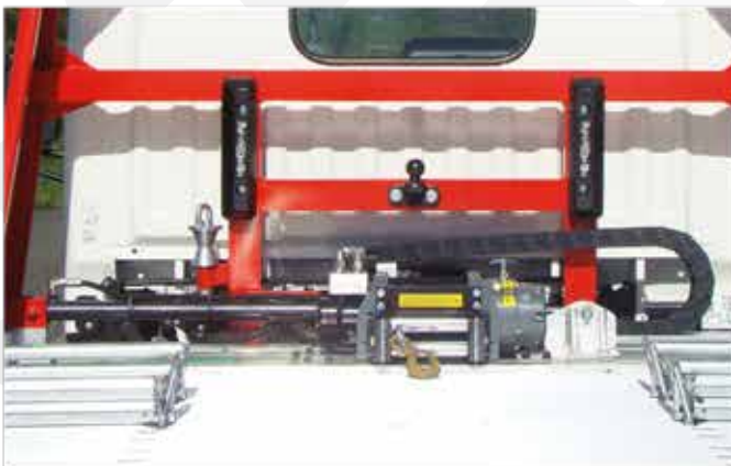
* Déplacement transversal hydraulique du treuil avec commande à distance radio.
